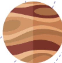
Jupiter
